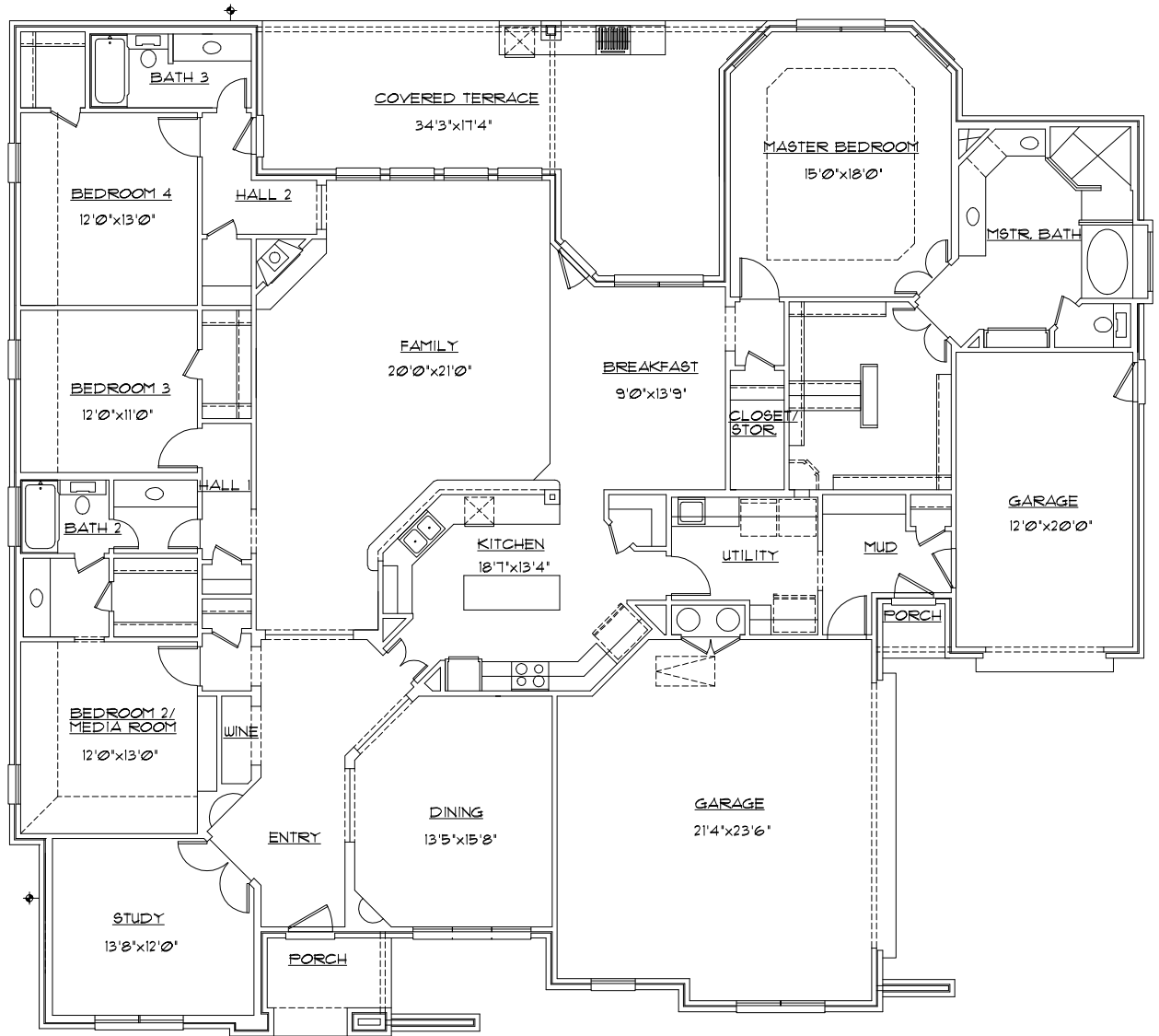
VAIL - FLOOR PLAN 4 BEDROOM / 3 BATH (3338#) 07094
